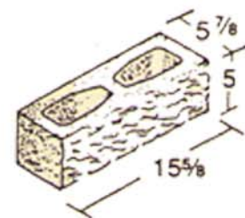
6 x 5 x 16
