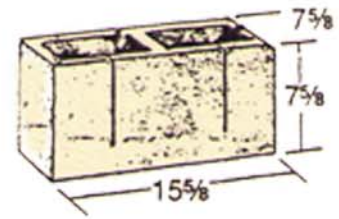
8 x 8 x 16 Type A-1
